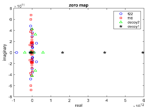
شکل ۲۱: الگوی قرارگیری صفرهای جنگنده‌ها و دکوی‌ها به صورت RMSE تطبیقی
