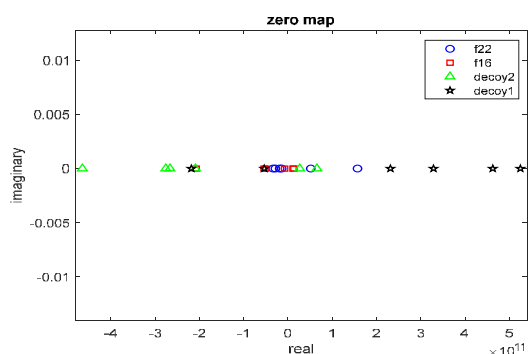
شکل ۲۳: الگوی قرارگیری صفرهای جنگنده‌ها و دکوی‌ها به صورت RMSE ثابت
