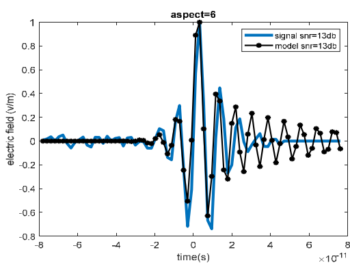
شکل ۱۸: سیگنال دریافتی از سمت پایین دکوی ۱ در حوزهی زمان به صورت RMSE ثابت
