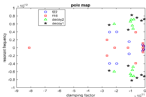
شکل ۲۲: الگوی قرارگیری قطبهای جنگنده‌ها و دکوی‌ها به صورت RMSE ثابت
