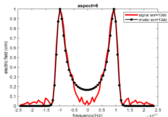
شکل ۱۷: سیگنال دریافتی از سمت پایین دکوی ۱ در حوزهی فرکانس به صورت RMSE تطبیقی
