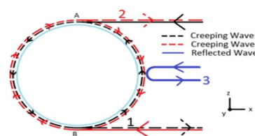
شکل ۲: بازتاب آینه‌ای و امواج خزنده‌ی سطحی از اجسام کروی و استوانه‌ای [۵، ۹]
