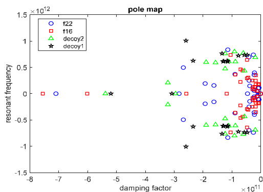
شکل ۲۰: الگوی قرارگیری قطبهای جنگنده‌ها و دکوی‌ها به صورت RMSE تطبیقی
