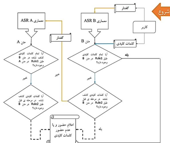
شکل ۶: فرآیند واژه‌یابی
