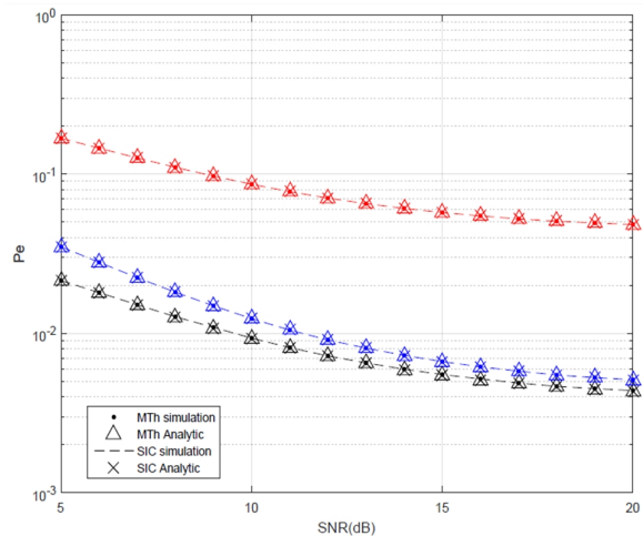
شکل (۵): منحنی‌های شبیه‌سازی و تحلیلی احتمال خطا بر حسب SNR(dB) برای آشکارسازهای MTh و SIC در حالت A_1\bar{h}_1 > A_2\bar{h}_2 + A_3\bar{h}_3 با مقادیر k = 17 \text{ dB} و A_1 = 6, A_2 = 3, A_3 = 1
