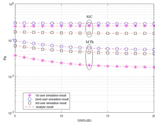
شکل (۶): منحنی‌های شبیه‌سازی و تحلیلی احتمال خطا بر حسب SNR(dB) برای آشکارسازهای MTh و SIC در حالت A_1\bar{h}_1 < A_2\bar{h}_2 + A_3\bar{h}_3 با مقادیر k = 17 \text{ dB} و A_1 = 9, A_2 = 6, A_3 = 4
