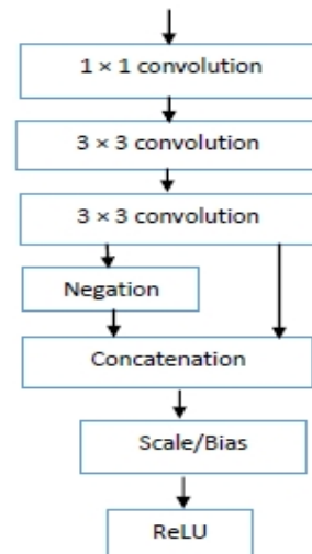
شکل ۲: ساختار 3 \times 3 i.ReLU پیشنهادی
