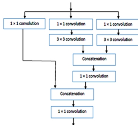
شکل ۳: ساختار inception i.inception پیشنهادی
